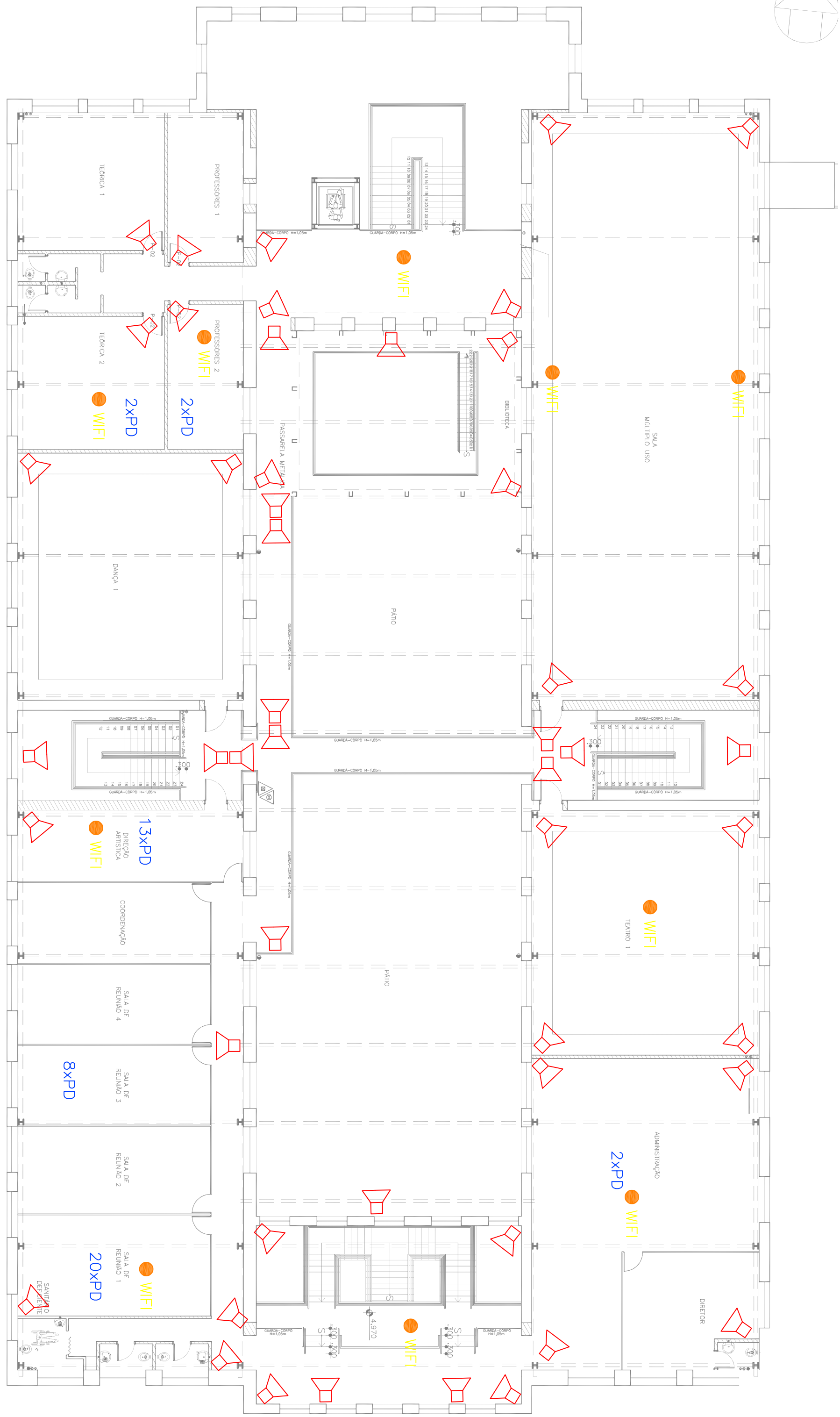
Planta 3º Pavimento ESC: 1:100
